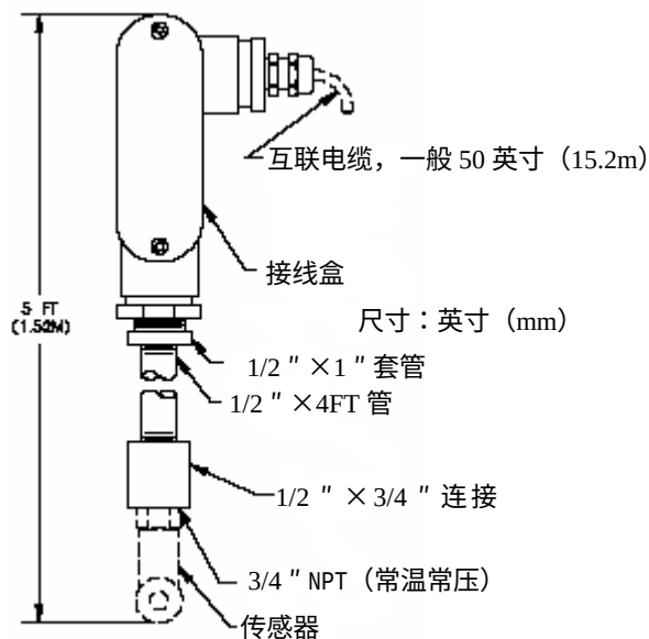
图2-1 液浸安装说明
