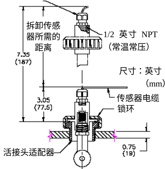
图 2-3 法兰安装说明
