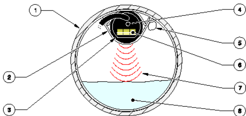
图 37 管道端视图
