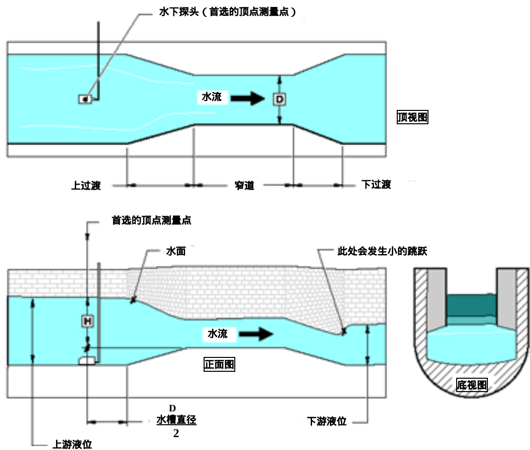
图 53 Leopold-Lagco 型水槽
